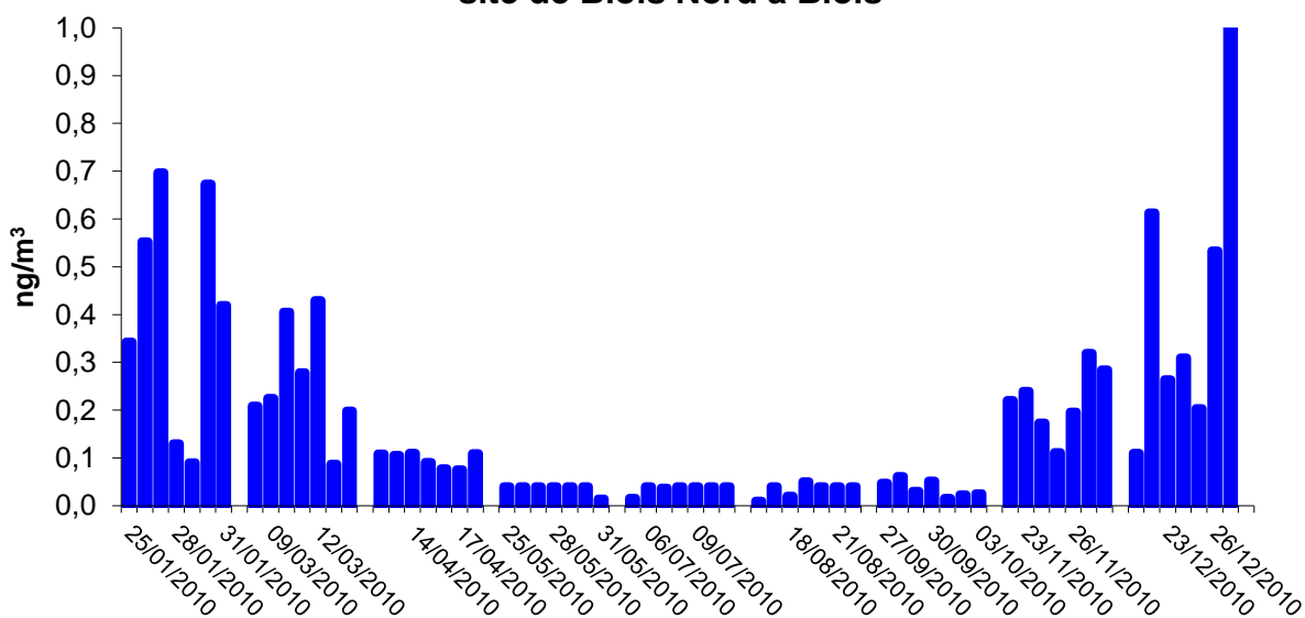
Evolution des concentrations Benzo(a)pyrène en 2010 sur le site de Blois Nord à Blois
