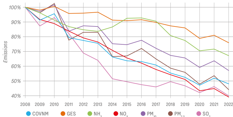
Figure 5 : Évolution annuelle des émissions polluantes depuis 2008 en région Centre-Val de Loire (base 100 en 2008).
