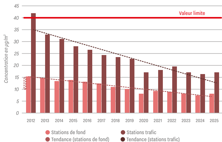
Figure 7 : Évolution des moyennes annuelles en NO 2 .
