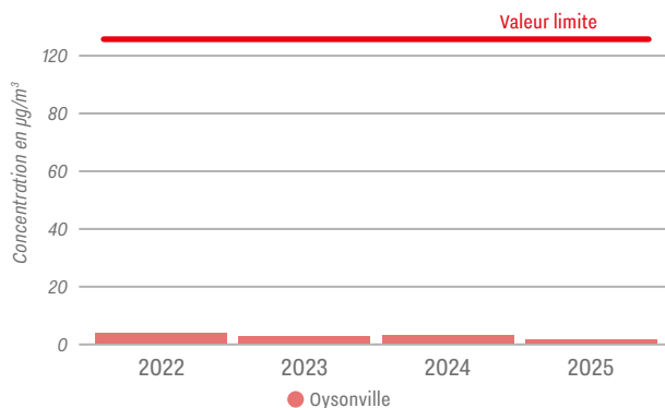
Figure 13 : Évolution annuelle des maxima journaliers en \text{SO}_2 à Oysonville.
