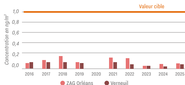
Figure 15 : Évolution des moyennes annuelles en benzo(a)pyrène sur la région Centre-Val de Loire de 2016 à 2025.
