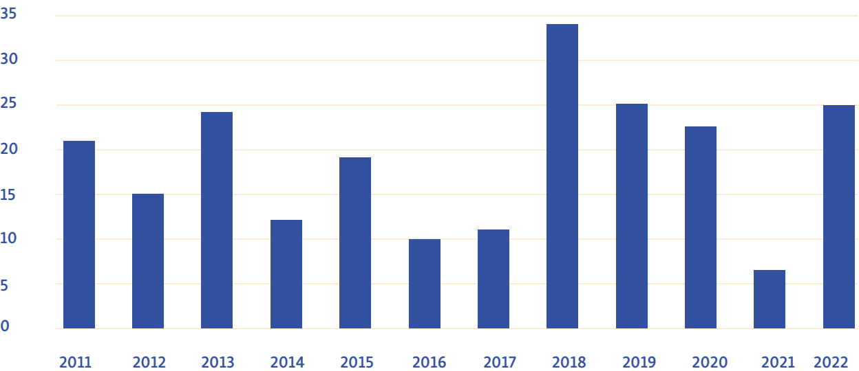
Figure 11: Nombre de jours de dépassement de 120 µg/m³ sur 8 heures pour l’ozone depuis 2011
