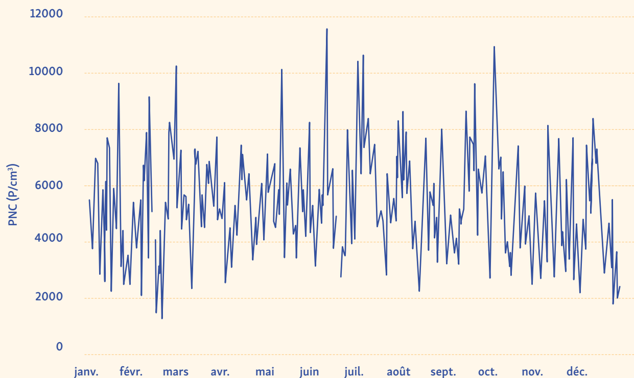
Figure 22: Concentration totale en nombre (PNC) journalière mesurée en 2022 à La Source-CNRS
